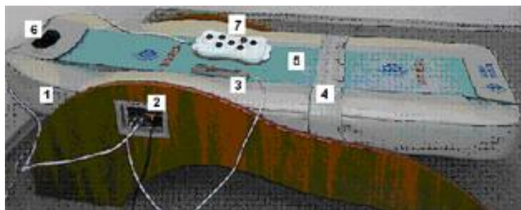
Рис. 1. Общий вид термомассажного ложа SAMMI SM-6000.
