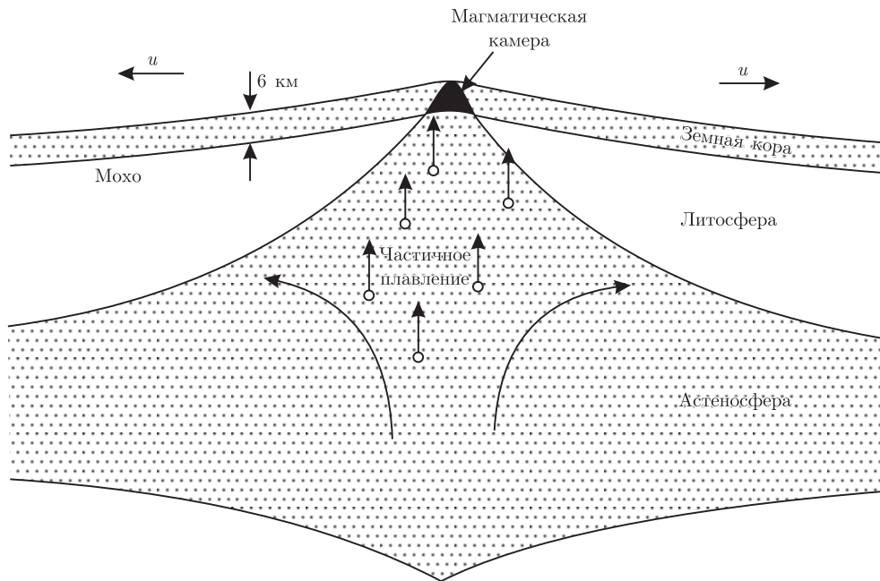
Рис. 2. Схема раздвигания плит и наращивания океанической земной коры в процессе вдавливания астеносферного материала в ослабленные зоны в областях срединных океанических хребтов
