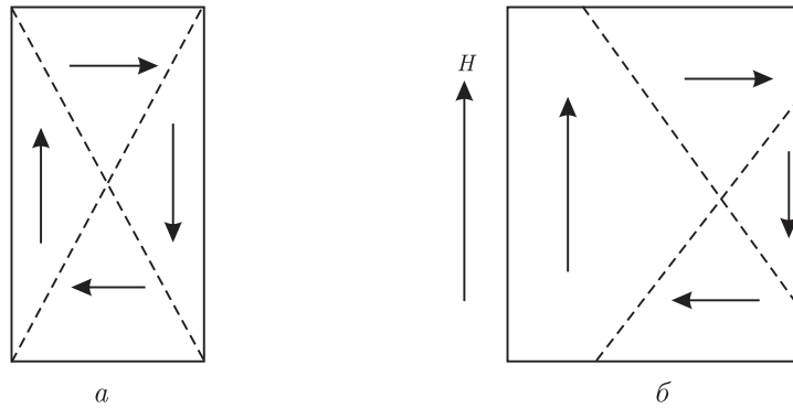
Рис. 1. Распределение энергии, принимаемой и излучаемой доменами внутри объекта: a — при отсутствии потока внешней энергии; б — при наличии внешнего магнитного поля ( H )
