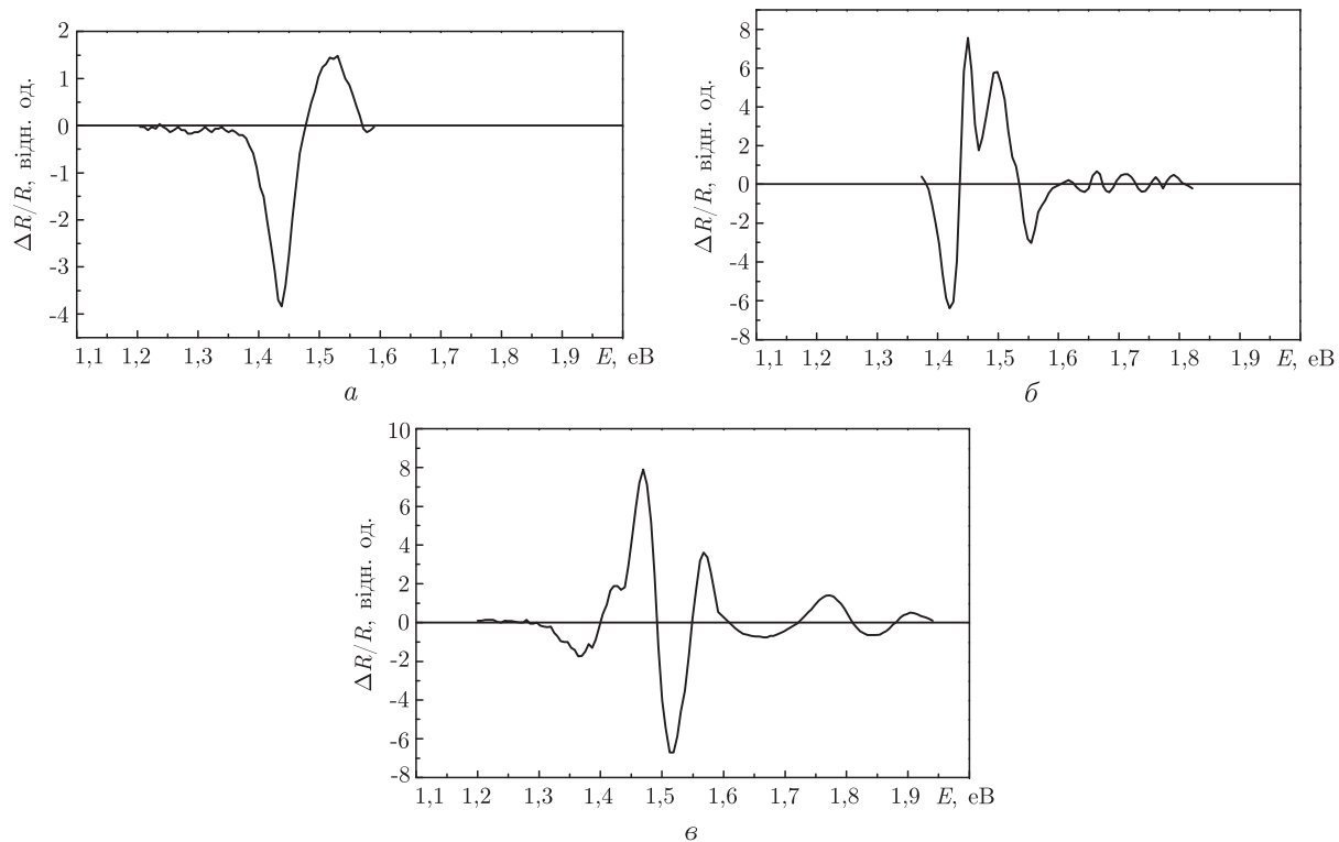
Рис. 1. Спектри електровідбивання поверхні GaAs до (а) і після її сульфидування протягом 5 (б) і 20 (в) хв
